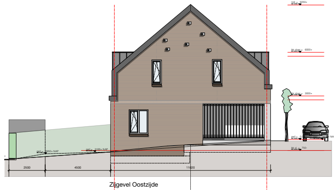
Zijgevel Oostzijde
