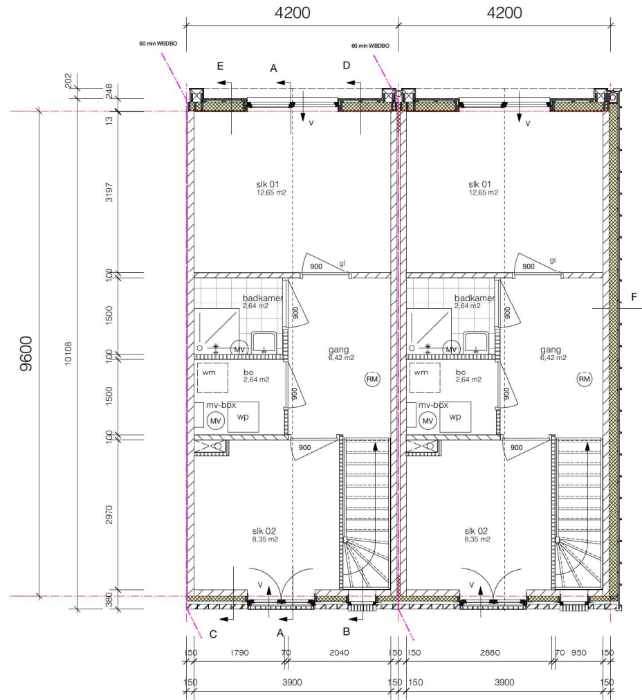
1e verdieping
