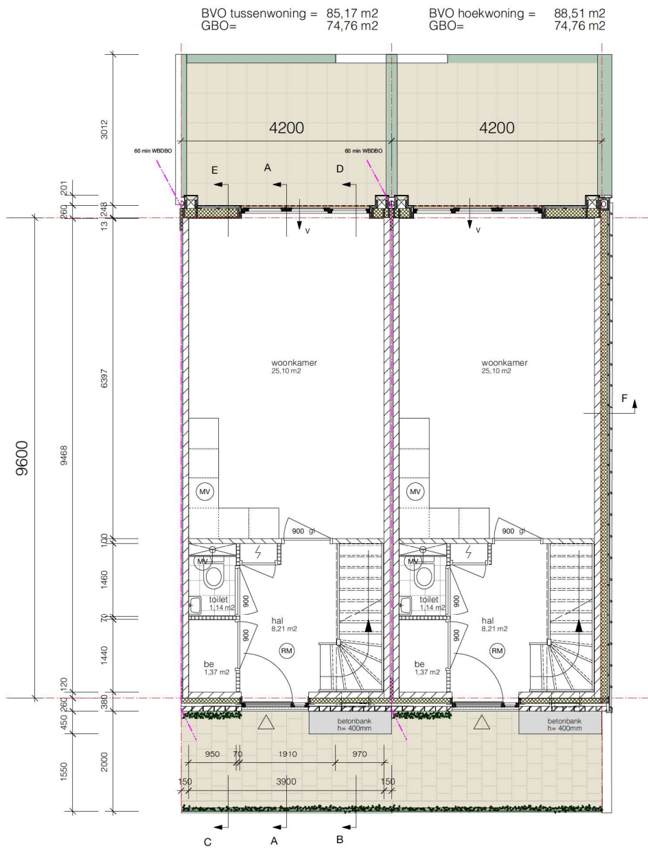
begane grond
