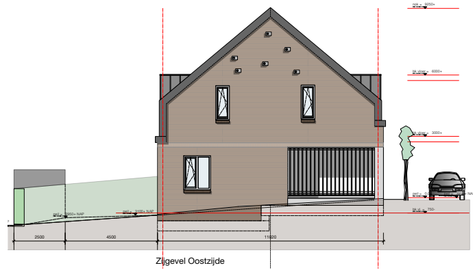
Zijgevel Oostzijde
